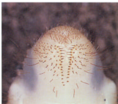
European chafer
