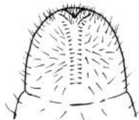
European chafer
